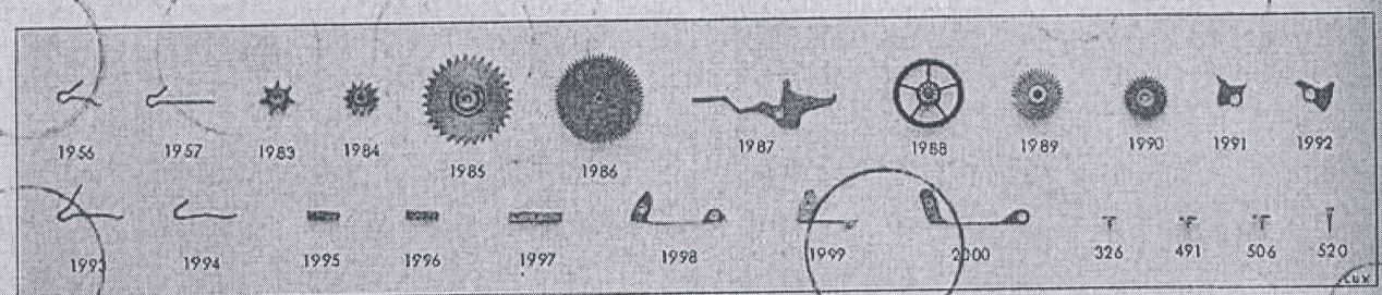
Calibre 217. — Supplément du cal. 215 pour Chronodato (chronographe avec quinquième).
